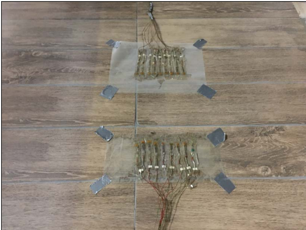
Abbildung A1: Prüfling mit Messfühlern
