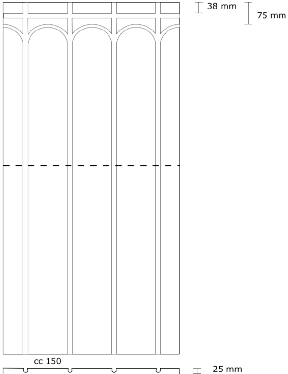
Abbildung A3: Systemaufbau
