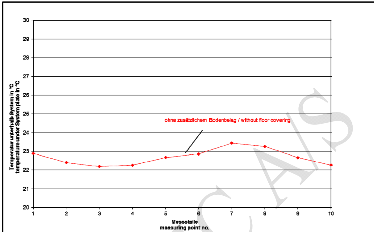
Abbildung A4: Temperaturen unterhalb Systemplatte
