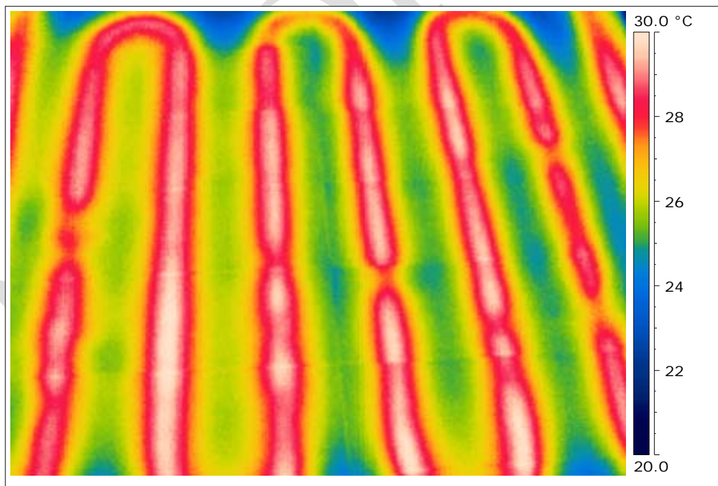
Abbildung A5: Thermographie Oberfläche
