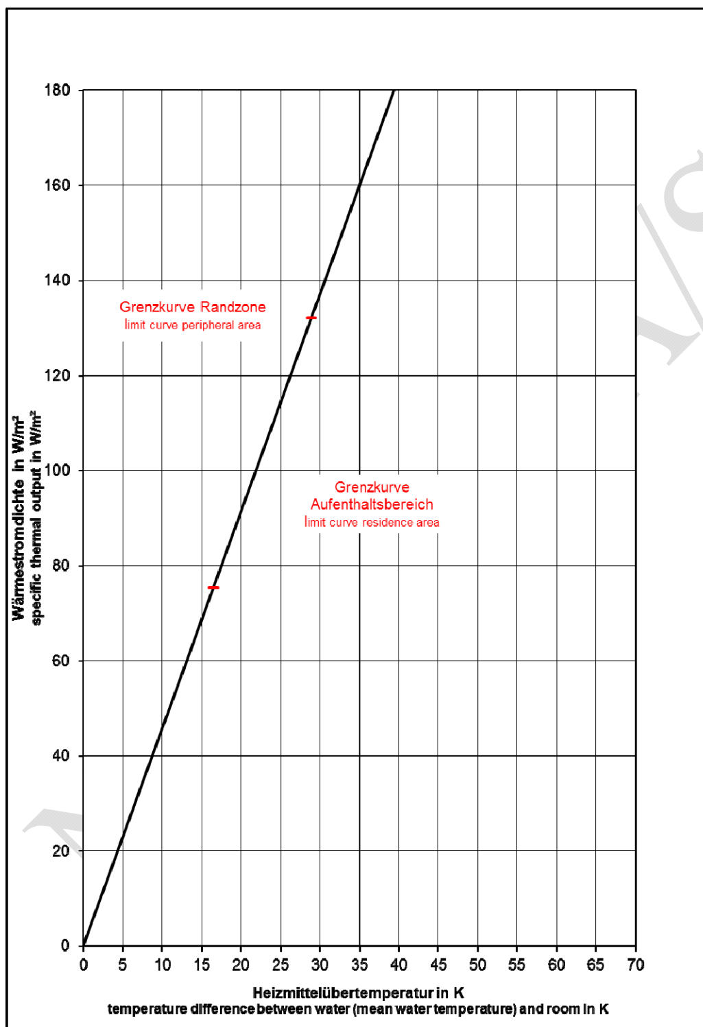
Abbildung 5: Leistungskennlinien Fußbodenheizungssystem
