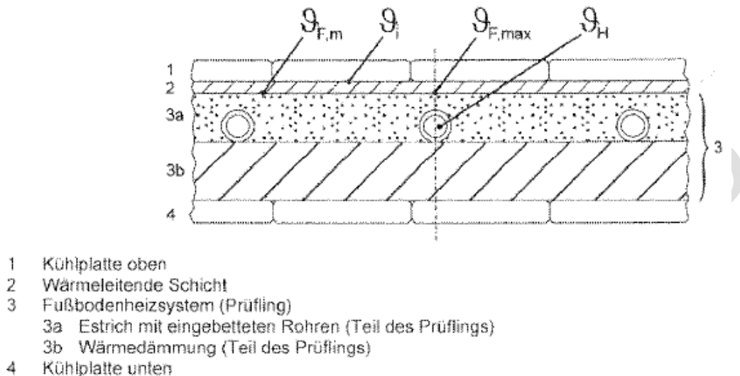
Abbildung 1: Prüfstand nach EN 1264 Teil 2 Abschnitt 9
